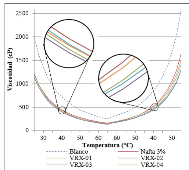
Fig. 2 Curvas de viscosidad con dosificación de 400 ppm
