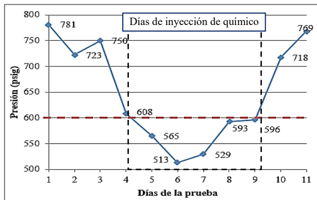
Fig. 7 Perfil de presión en la descarga de la bomba Booster
